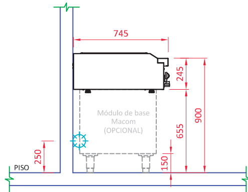
VISTA LATERAL
